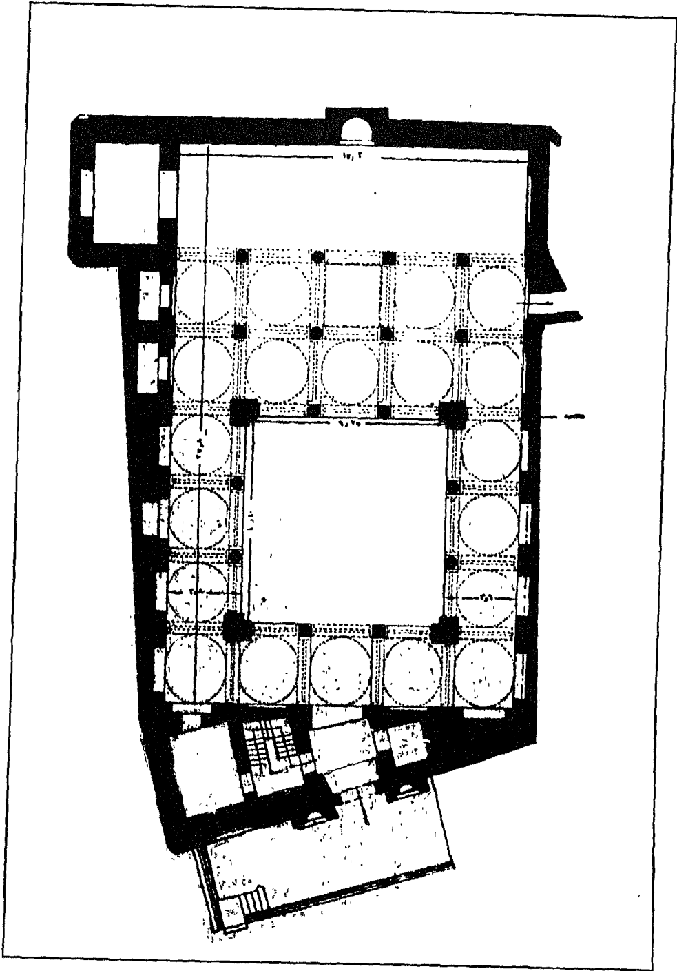
شكل (١٩) جامع الأقرم، مسقط أفقي عن أحمد فكري.
